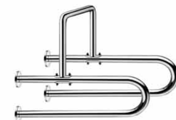
YX-3338 Material : SUS 304 Size(mm) : 600x650x500 Finish : Matt / Polish
