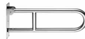
YX-3331 Material : SUS 304 Size(mm) : 600x280 Finish : Matt / Polish
