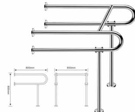
YX-3337 Material : SUS 304 Size(mm) : 800x800x800 Finish : Matt / Polish
